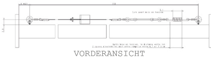
G130: Messung der Durchbiegung eines Balkens
