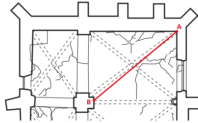
G20: Überwachung der Entwicklung des Abstands zwischen zwei Punkten, die mehrere Meter voneinander entfernt sind ("Auftrieb" von Bauwerken) mit Ableseung der Messung auf Augenhöhe und Aufzeichnung
